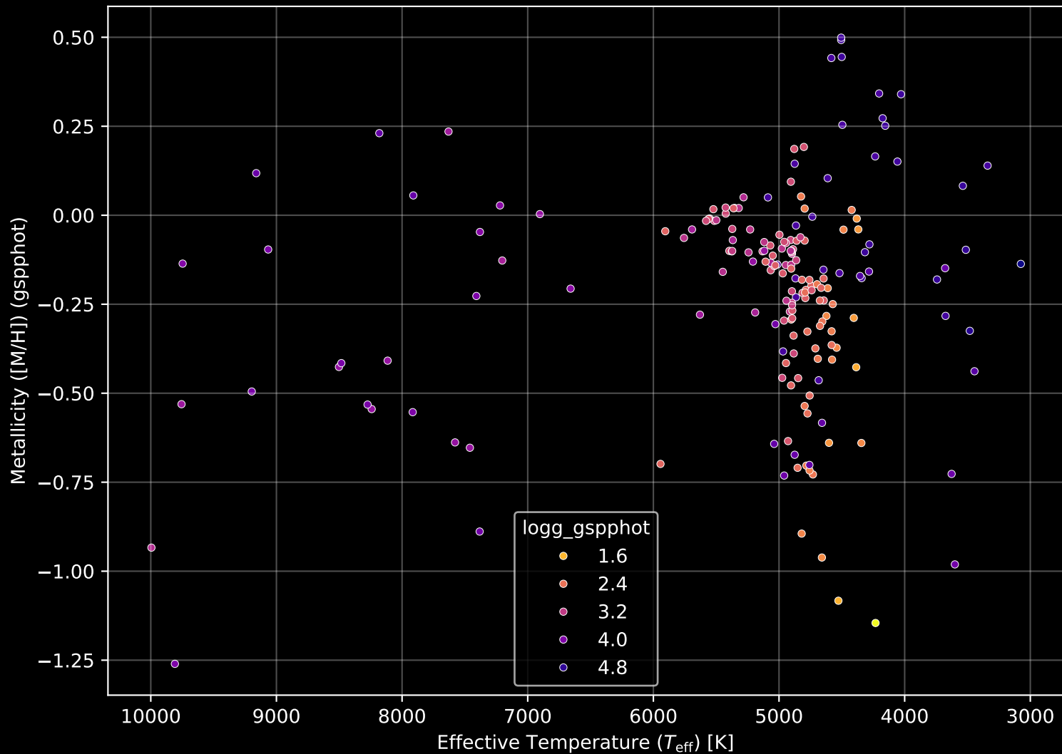
APOGEE DR17 Field: [188+18] Stellar Population Parameters (n= 190)
